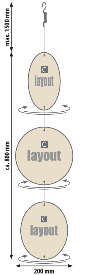
Produktansicht Deckenhänger
