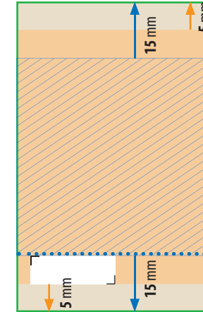
Perforation/Codierfeld Schmalseite
