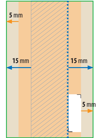
Perforation/Codierfeld Längsseite
