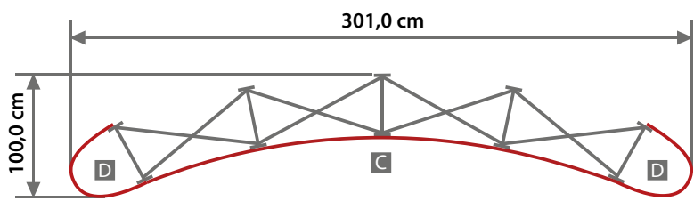
Systemabmaße
