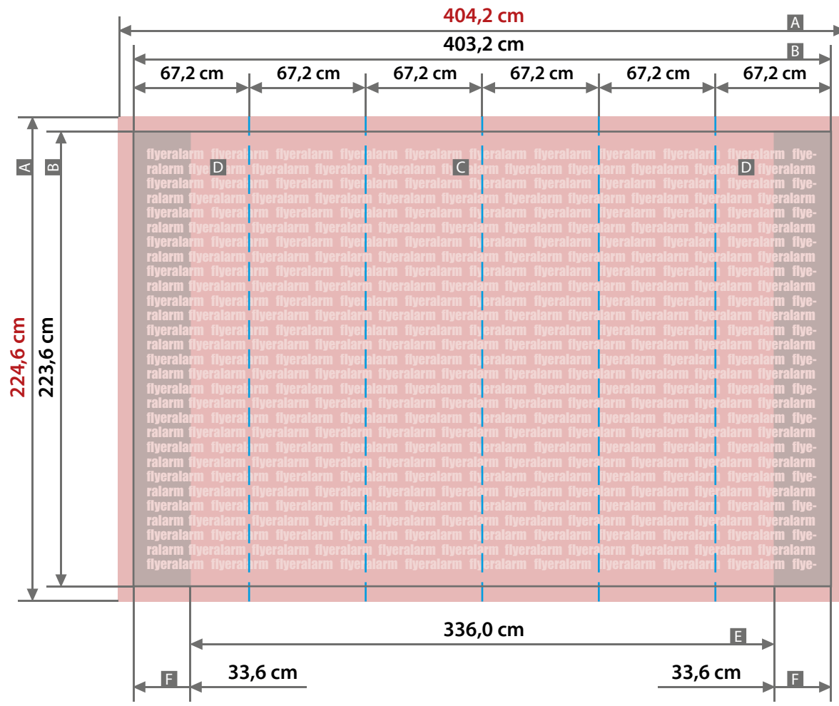
Systemabmaße
