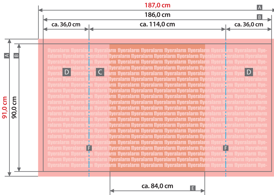
Darstellung Endformat - Druck mit Lamellenbahn verbunden
