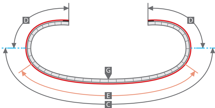
Darstellung Endformat - Druck mit Lamellenbahn verbunden
