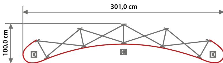
Systemabmaße
