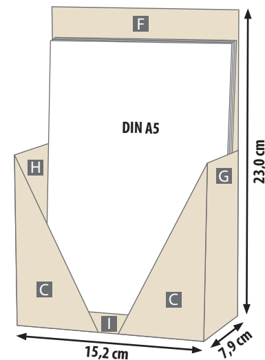
Produktansicht Kartenbox
