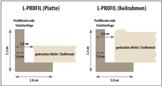
Schattenfugenrahmen im Querschnitt
